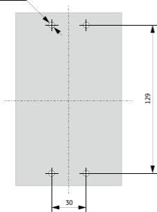
Разметка установочных отверстий
