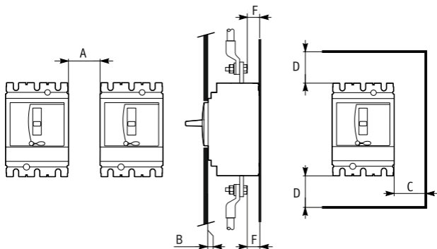
Рисунок 1 - безопасные расстояния при установке в шкафу НКУ
