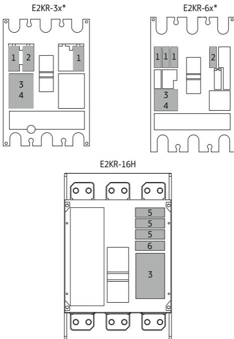
Рисунок 2 - схема установки дополнительных устройств. На рисунке обозначены:
