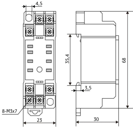
Розетка для RI-52
