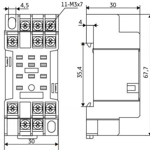
Розетка для RI-53
