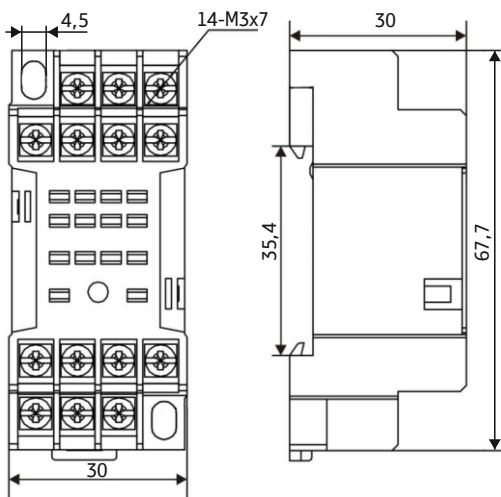
Розетка для RI-54
