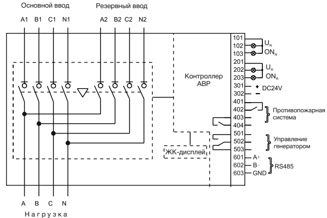
Рис. 6. Схемы подключения: 6а - базовый тип; 6б - универсальный тип
