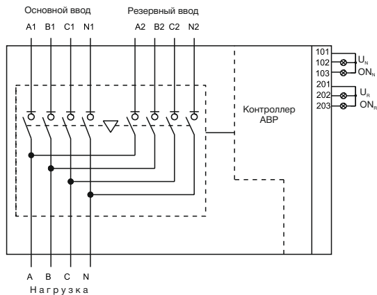
Рис. 6. Схемы подключения: 6а - базовый тип; 6б - универсальный тип
