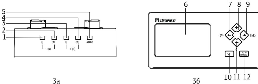
Рис. 3. Лицевая панель контроллера: 3а - базовый тип; 3б - универсальный тип
